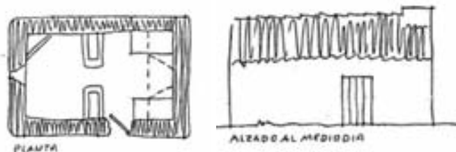
Planta y Alzado de una quintería Bocetos, MIGUEL FISAC
